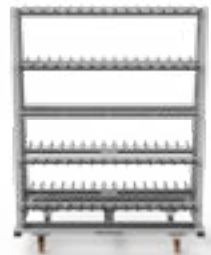
Carr 200 Q / Carr 300 Q Carro de transporte y almacenamiento perfiles en posición vertical Carr 200 Q Anchura: 912 mm - Longitud: 1282 mm. Carr 300 Q Anchura: 912 mm - Longitud: 1718 mm. Superficies de contacto revestidas en material plástico antirraya y antichoque.
